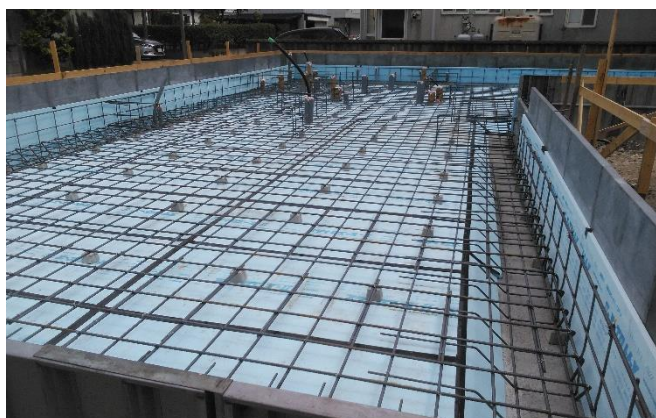
配筋の状況
